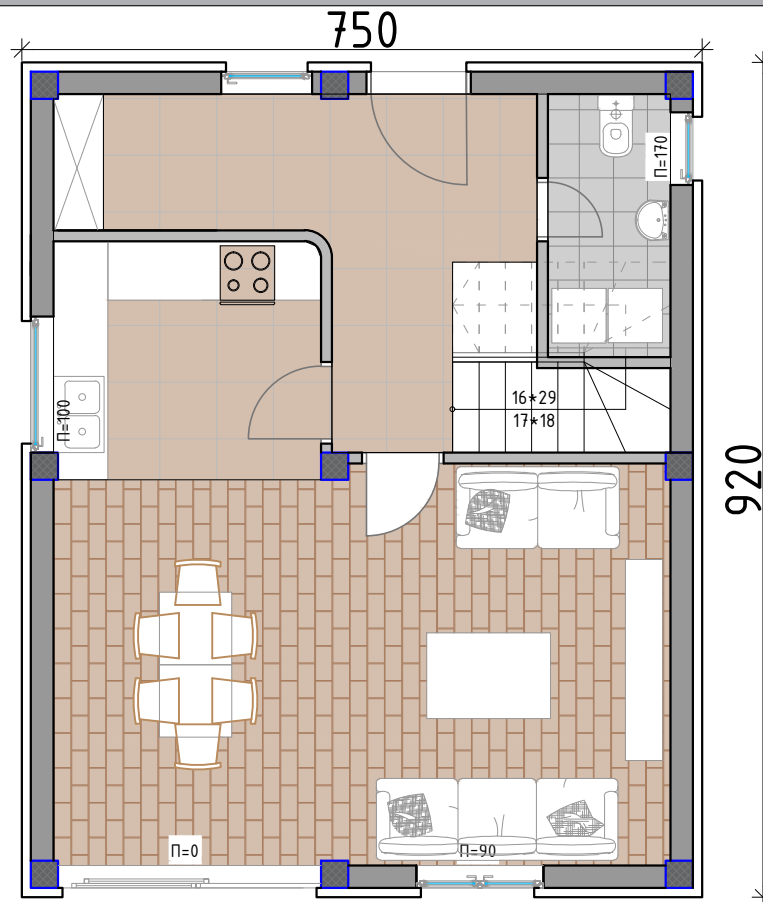
ОСНОВА НА ПРИЗЕМЈЕ
